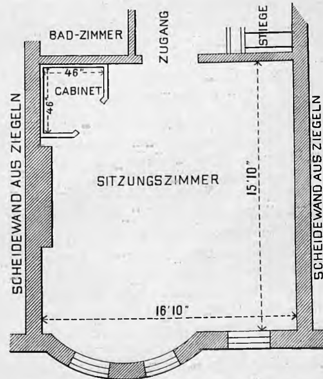
Grundriss des Sitzungs-Zimmers der Fran Fay.
